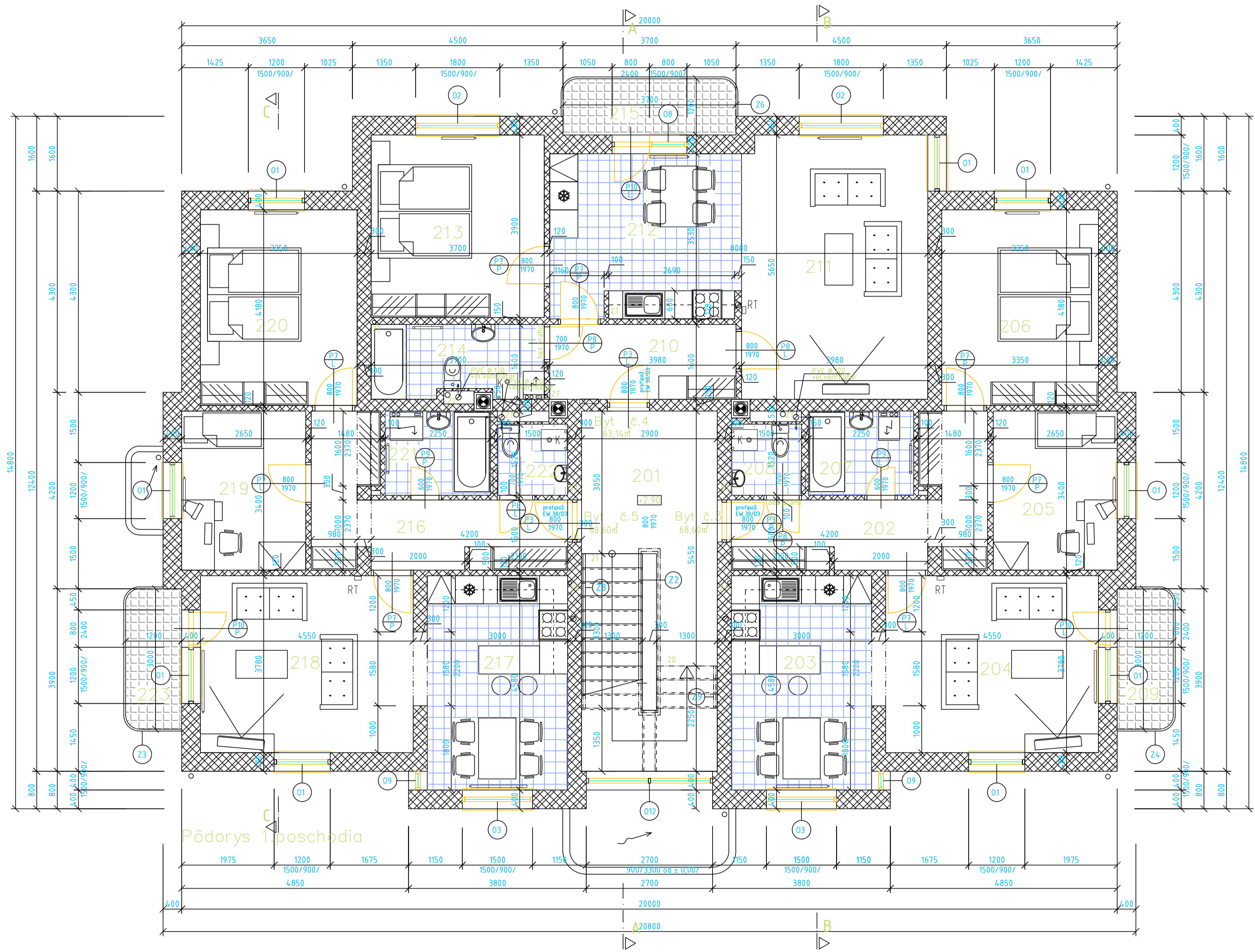
Pôdorys 1.poschodia
